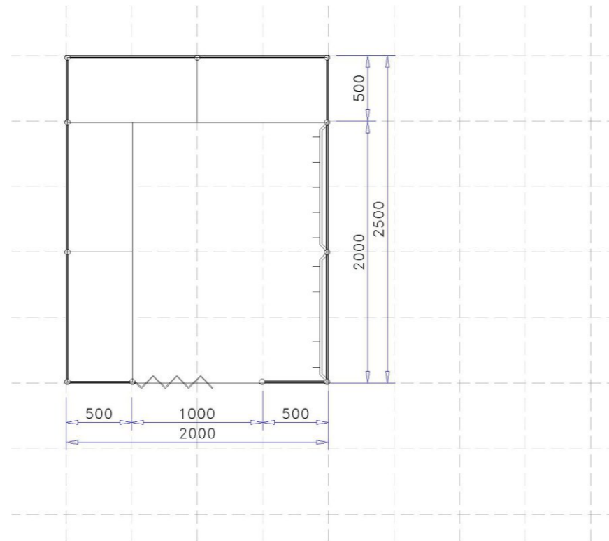
SKLAD S3 - PŮDORYS
