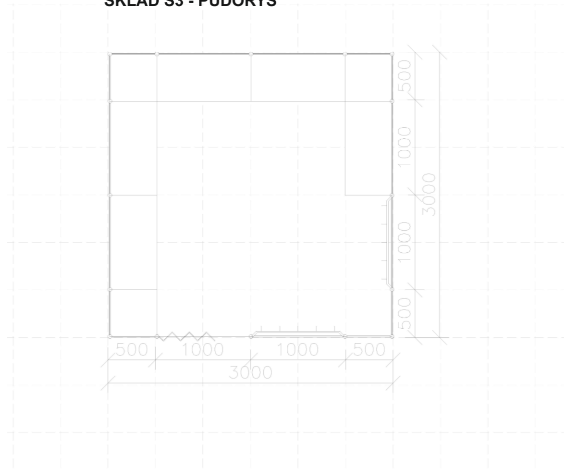
SKLAD S3 - PŮDORYS
