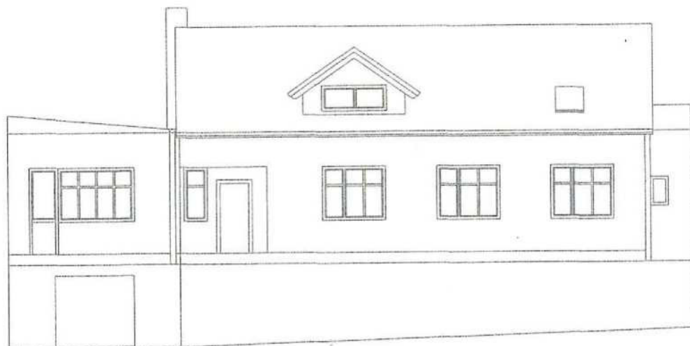
POHLED JIŽNÍ
