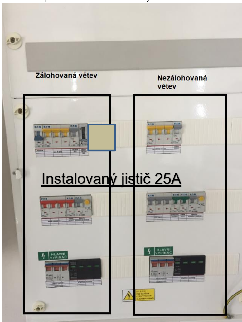
Obr.4 Rozvaděč s možností instalace jištění PEGAS
