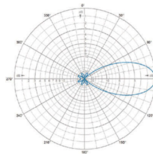
E-Plane | 425 MHz
