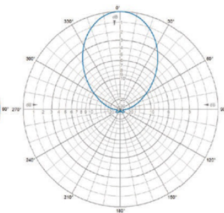
H-Plane | 425 MHz
