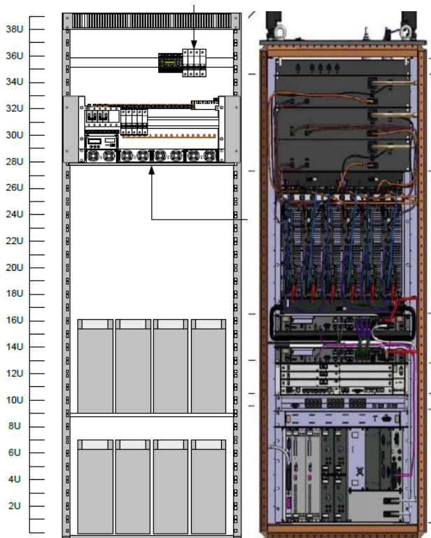
Obr. 3 sestava technologie
