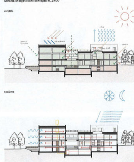
Schéma energetického konceptu m_1400
