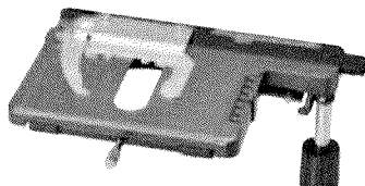
XY stolek s keramickým povrchem a držákem 2 preparátů
