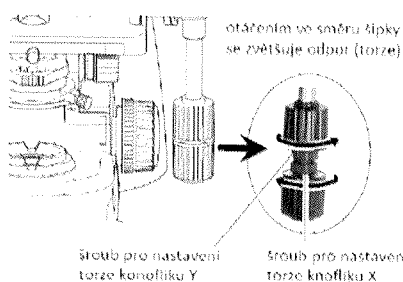
nastavení odporu proti otáčení (torze) knoflíků X a Y
