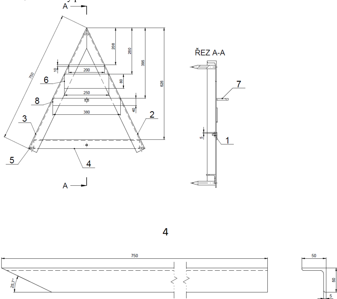
obr. č 8 – Rozměry podstavce
