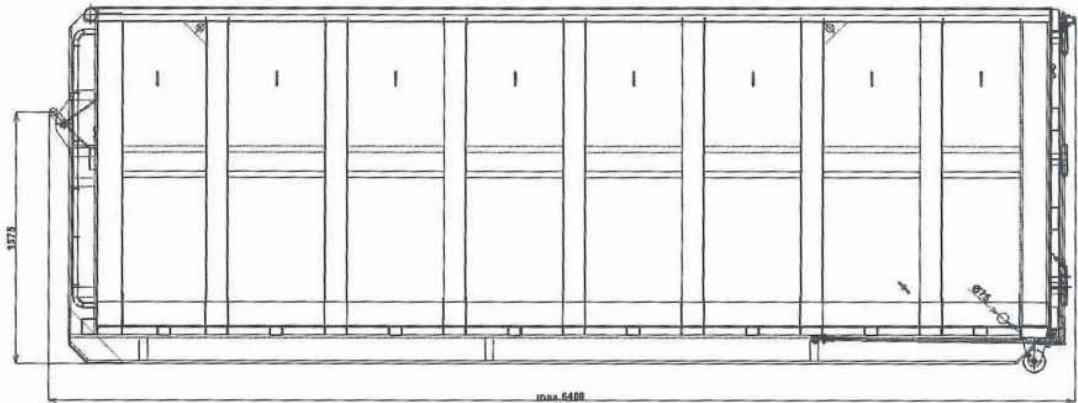
levá strana
