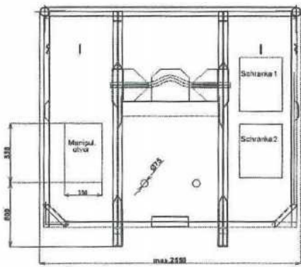
přední pohled
