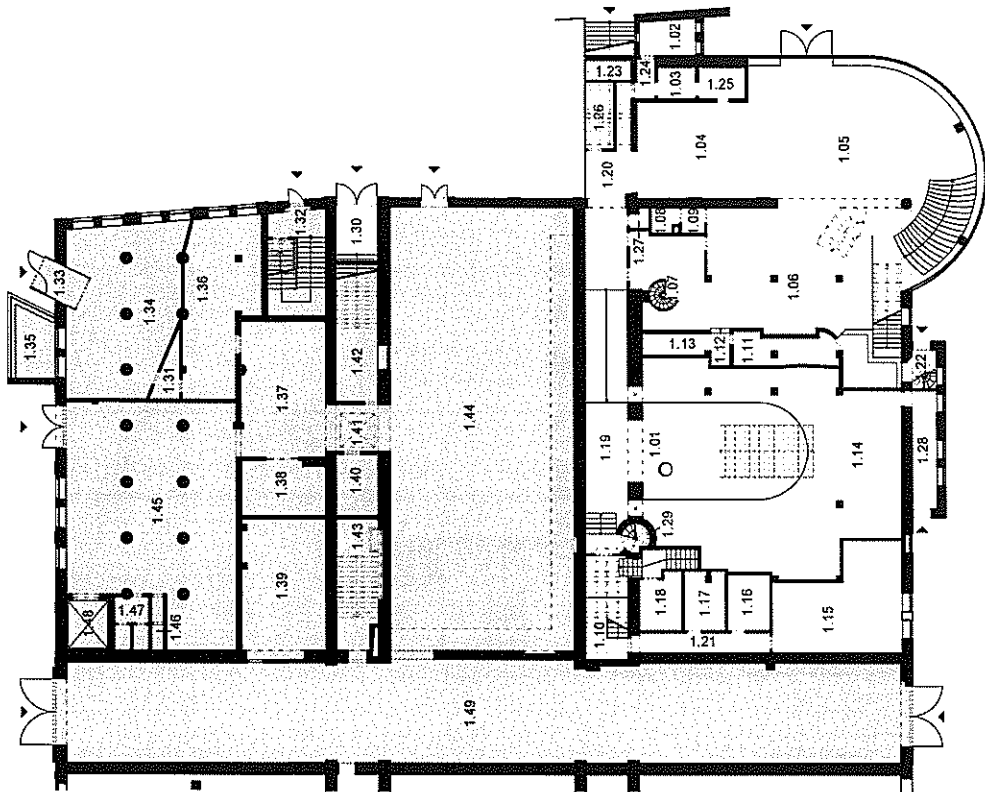
Schematický půdorys 1.NP
