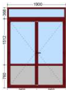
ven otvíravé vnější pohled (exteriér)
