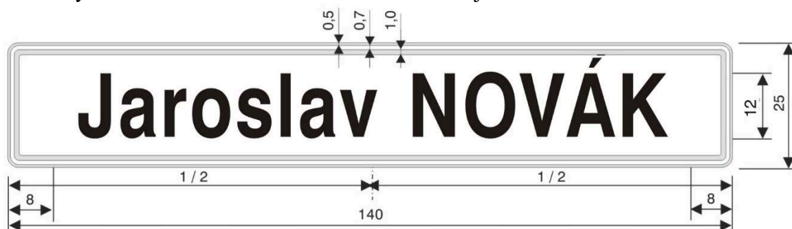
Rozměrové nákresy rámečků
