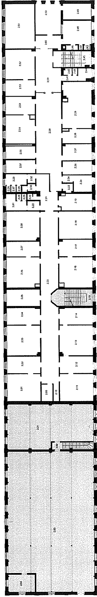
Schematický půdorys ZNP
