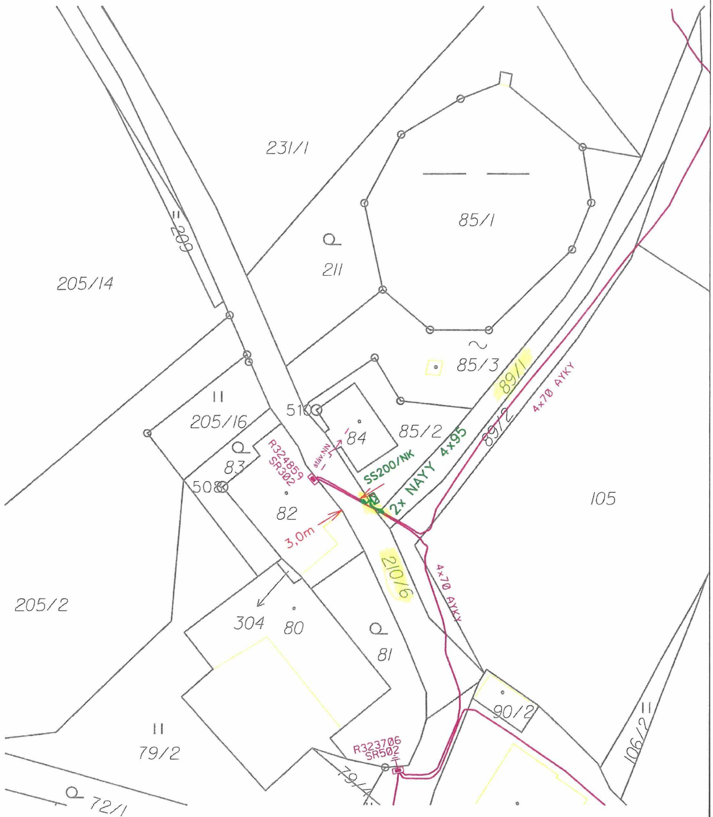
ULOŽENÍ KABELU NN V CESTĚ - PŘEKOP
