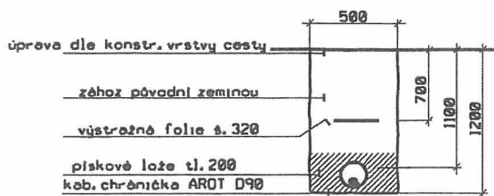
ULOŽENÍ KABELU NN V CESTĚ - PŘEKOP
