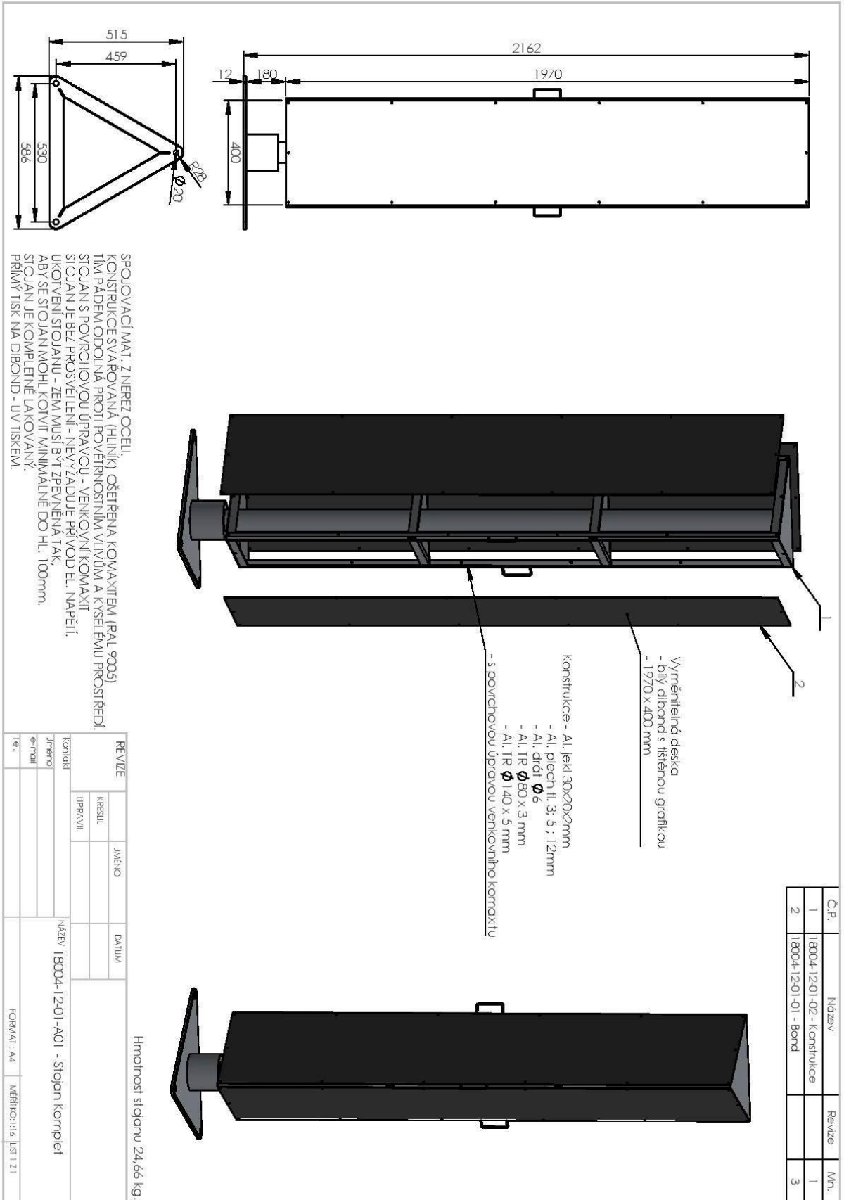
Příloha č. 1: projektová dokumentace k informačnímu panelu
