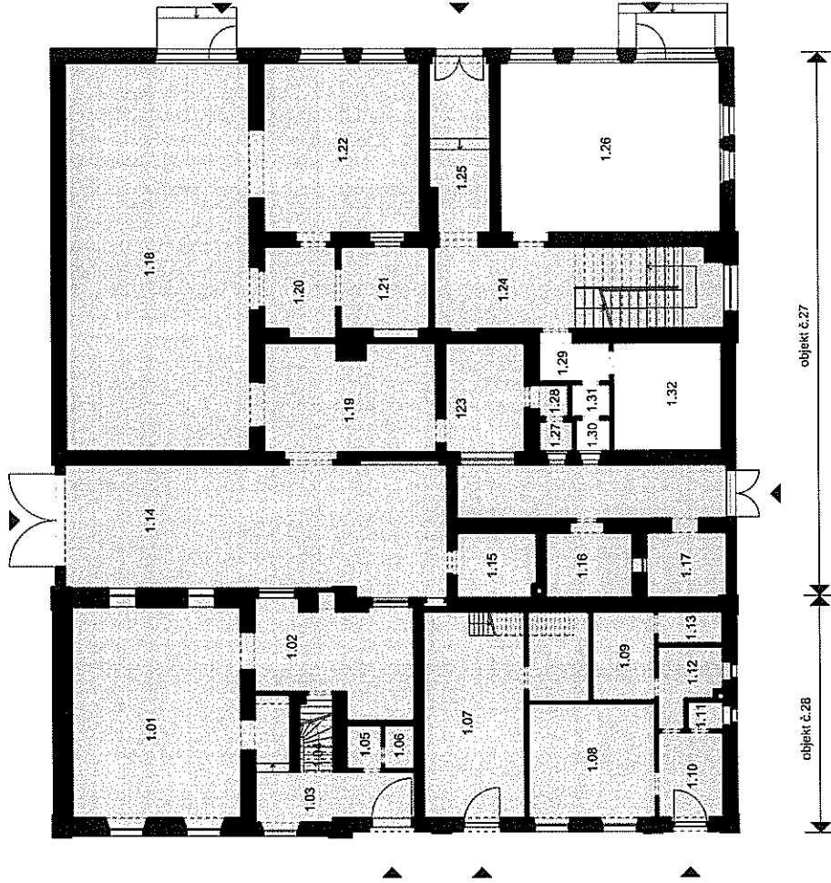
Schematický půdorys 1.NP
