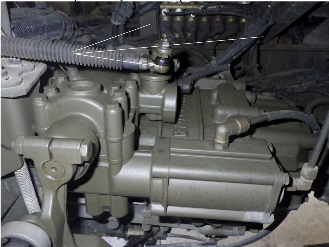
Foto č. 2 – lanovody k řazení rychlostních stupňů
