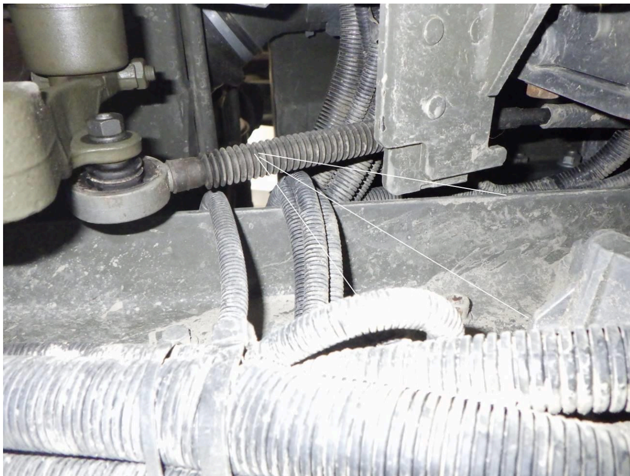
Foto č.3 – posilovač spojky
