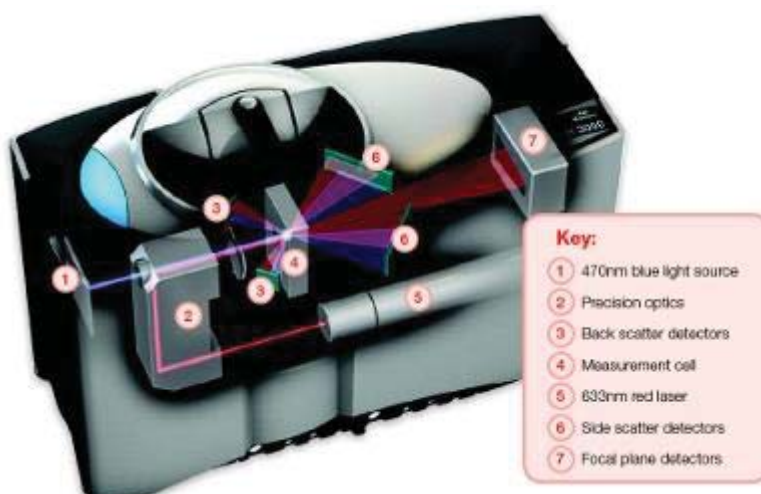
Obr.1 Optická lavice Malvern MS-3000
