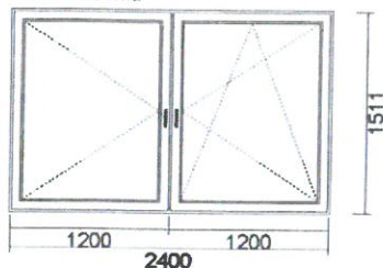
19) OKNO 2-KŘ (O+OS) (PEV.SL.) 2400x1511
