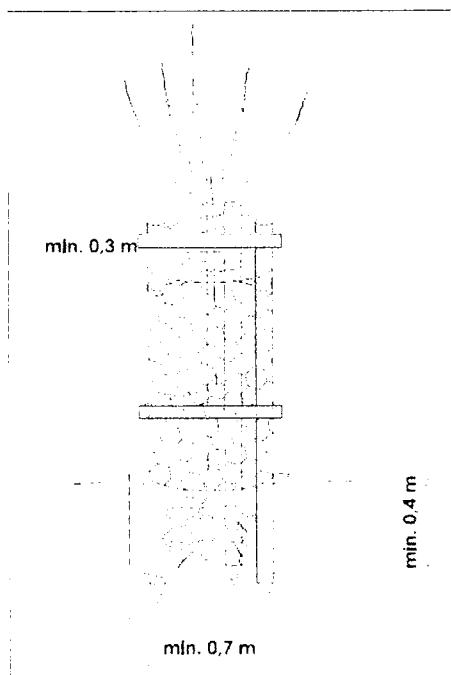
Obr. č. 3. – Třibodový systém kotvení a ochranný plášť
