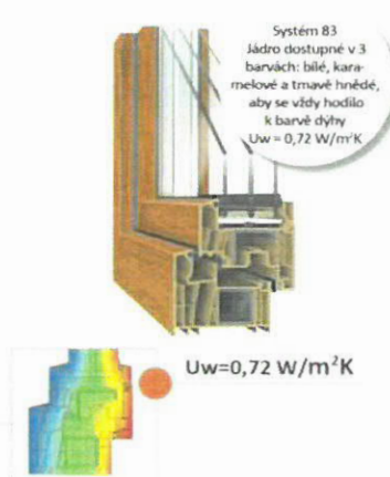
Trojité prosklení 48 mm Distanční rámeček SWISSPACER V, argon
