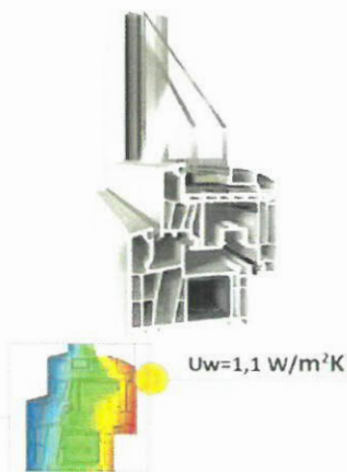
Dvojitě zasklení 24 mm Hliníkový distanční rámeček
