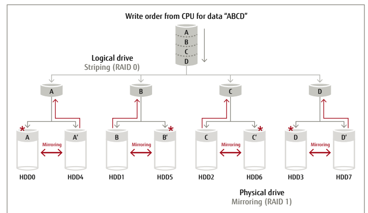
RAID 1+0
