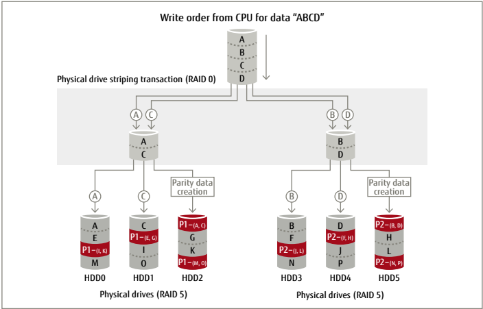
RAID 5+0
