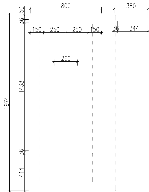
AT Š 1ks Šatní stěna 800x1974x380mm deska LTD 573 dub mahorn PLUS tl. 36mm ukotvení na zeď 5x věšák Livorno nikl matný 35611 pevné police
