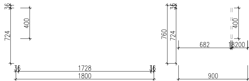
AT S3 1ks Kancelářský stůl 1800x760x900mm konstrukce LTD 573 dub mahorn PLUS tl. 36mm lub tl.18mm
