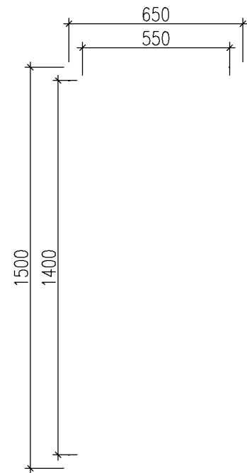
AT Z 3ks Zrcadlo 650x1500x18mm deska LTD 573 dub mahorn PLUS tl. 18mm ukotvení na zeď zrcadlo 550x1400mm
