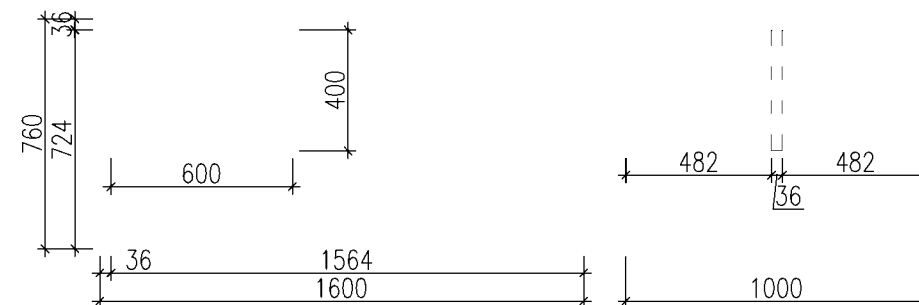
AT P3 1ks Přístavba ke stolu 1600x760x1000mm konstrukce LTD 573 dub mahorn PLUS tl. 36mm
