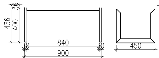
AT M 6ks Konferenční stůl 900x450x436mm deska LTD 573 dub mahorn PLUS tl. 36mm podnoží Mobi-q
