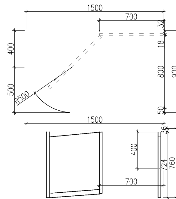
AT ZS2-L 2ks Rohový díl zasedacího stolu LEVÝ 1500x760x900mm deska LTD 573 dub mahorn PLUS tl. 36mm lub tl. 18mm podnoží Mobi-q
