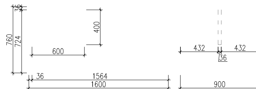
AT P2 1ks Přístavba ke stolu 1600x760x900mm konstrukce LTD 573 dub mahorn PLUS tl. 36mm
