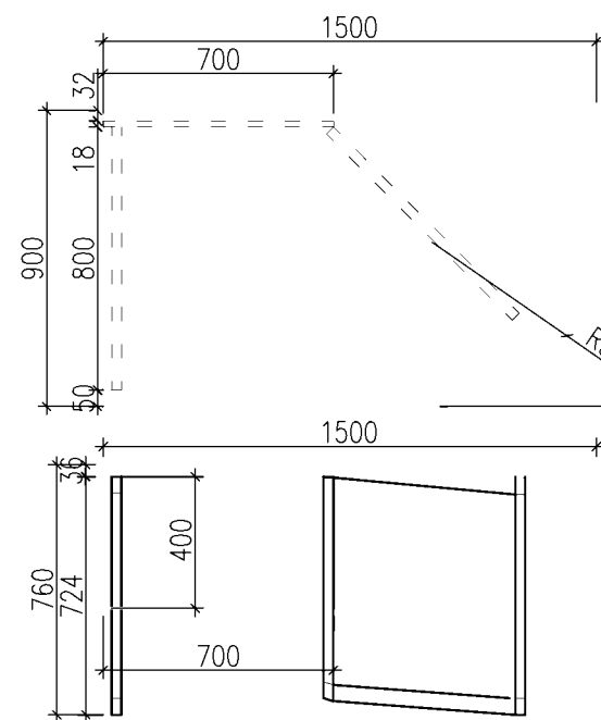
AT ZS2-P 2ks Rohový díl zasedacího stolu PRAVÝ 1500x760x900mm deska LTD 573 dub mahorn PLUS tl. 36mm lub tl. 18mm podnoží Mobi-q el. zásuvka 407831 otvor. 120mm
