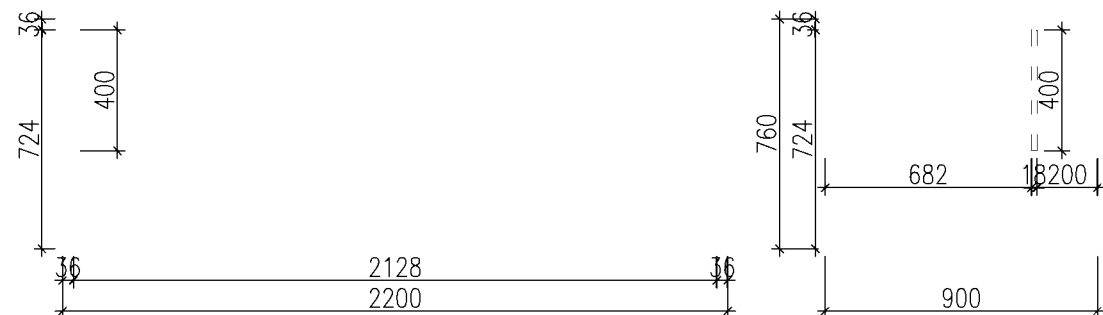
AT S1 4ks Kancelářský stůl 2200x760x900mm konstrukce LTD 573 dub mahorn PLUS tl. 36mm lub tl.18mm
