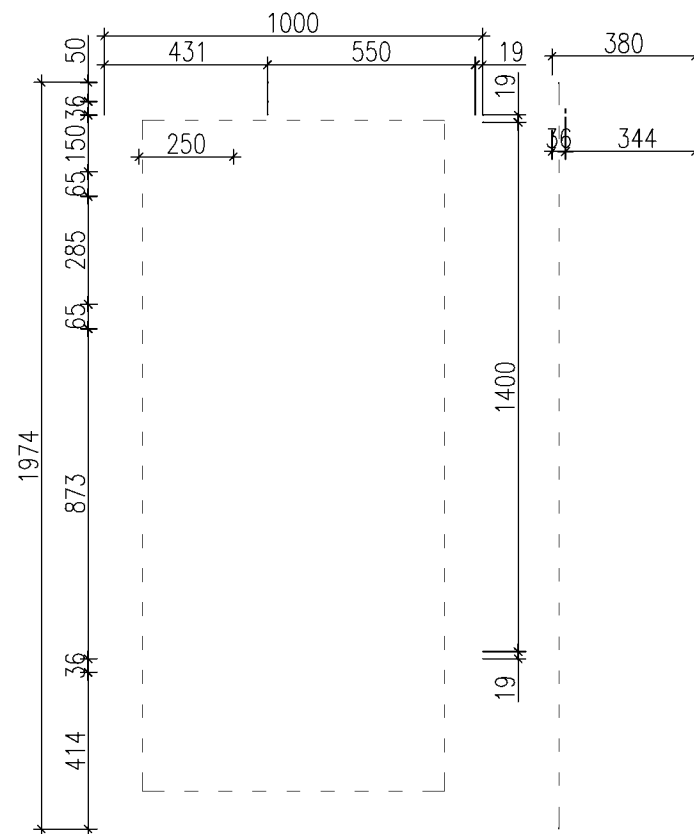
AT ŠZ 1ks Šatní stěna se zrcadlem 1000x1974x380mm deska LTD 573 dub mahorn PLUS tl. 36mm ukotvení na zeď 3x věšák Livorno nikl matný 35611 pevné police zrcadlo 550x1400mm
