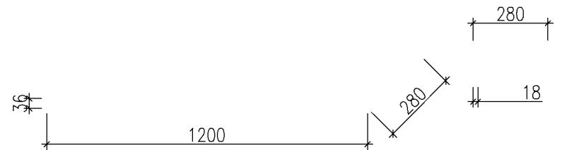
AT PO 1ks Nástěnná police 1200x36x280mm deska LTD 573 dub mahorn PLUS tl. 36mm ukotvení na zeď pomocí 4 trnů 15654+337998
