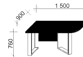
AT ZS2-P 2ks Rohový díl zasedacího stolu PRAVÝ 1500x760x900mm deska LTD 573 dub mahorn PLUS tl. 36mm lub tl. 18mm podnoží Mobi-q el. zásuvka 407831 otvor. 120mm
