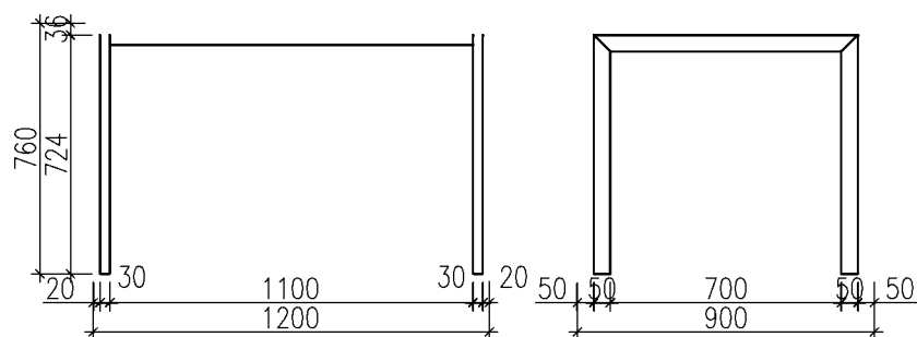
AT J2 1ks Jídelní stůl 1200x760x900mm deska LTD 573 dub mahorn PLUS tl. 36mm podnoží Mobi-q
