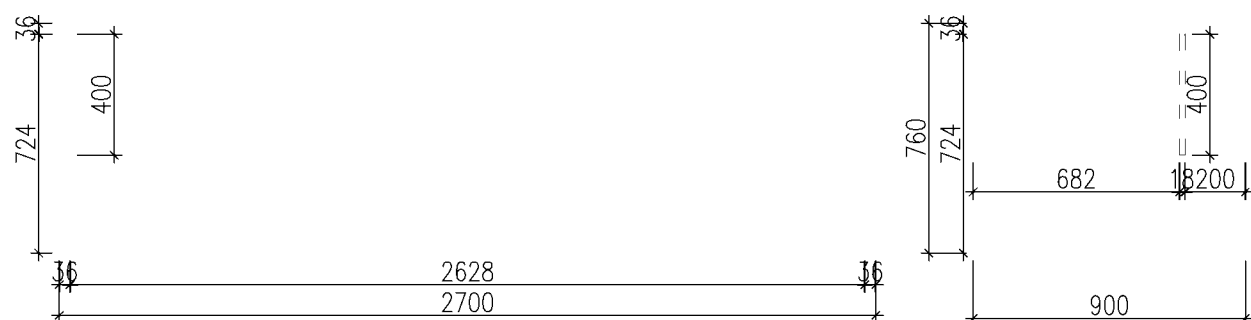
AT S2 1ks Kancelářský stůl 2700x760x900mm konstrukce LTD 573 dub mahorn PLUS tl. 36mm lub tl.18mm
