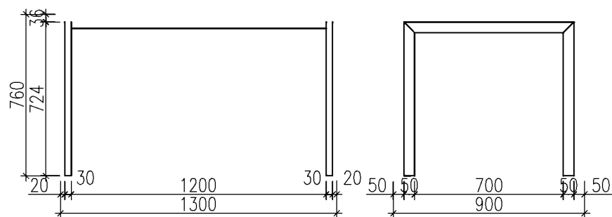
AT J1 1ks Jídelní stůl 1300x760x900mm deska LTD 573 dub mahorn PLUS tl. 36mm podnoží Mobi-q
