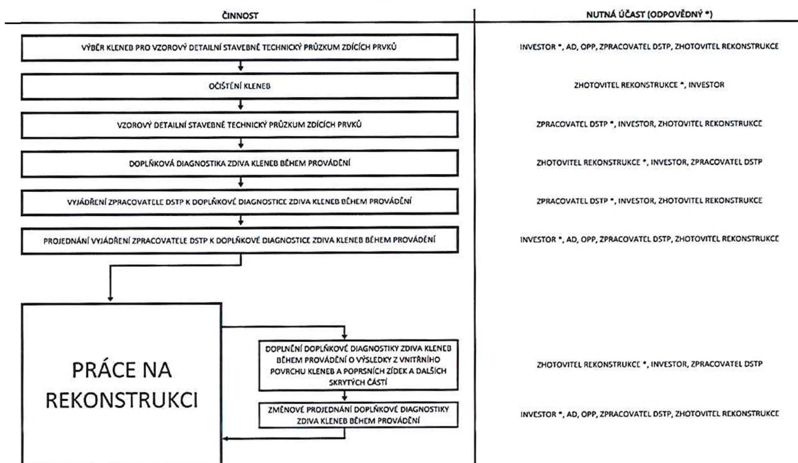
Obr. 1 Schéma průběhu doplňkového stavební technického průzkumu pro stavební objekty z pískovcového a žulového zdiva
