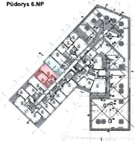
Půdorys 6.NP
