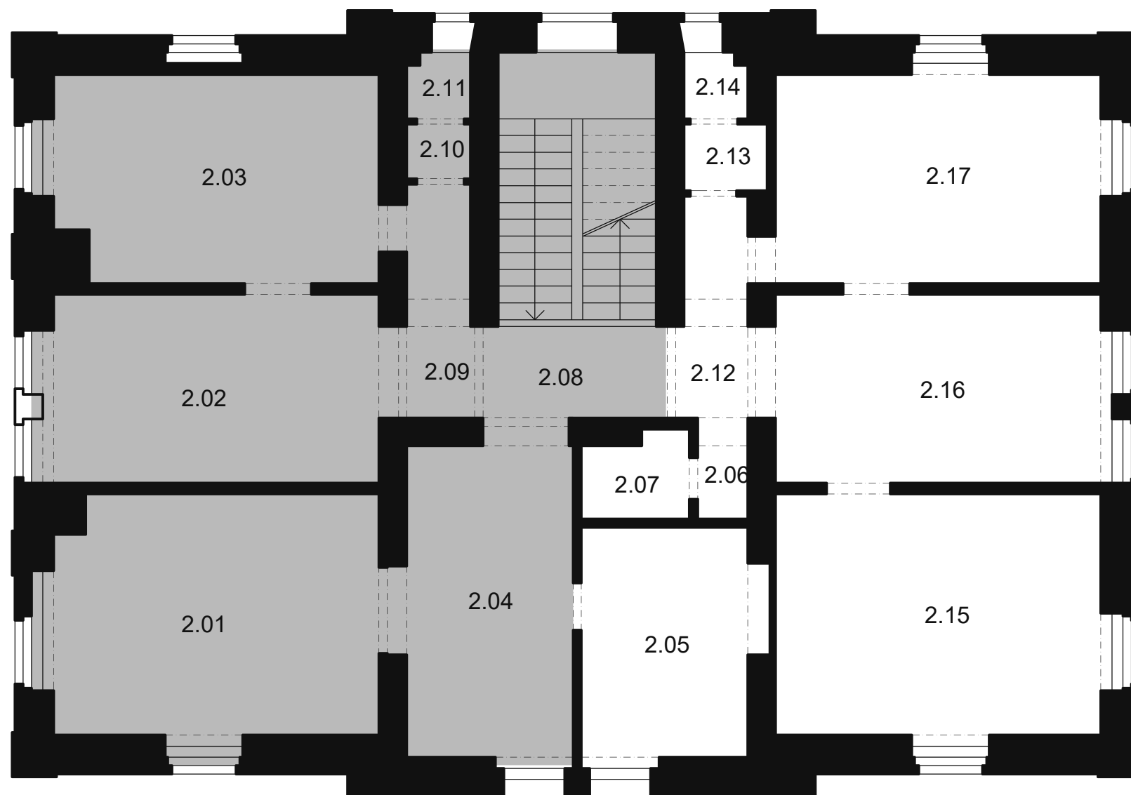
Schematický půdorys 2.NP
