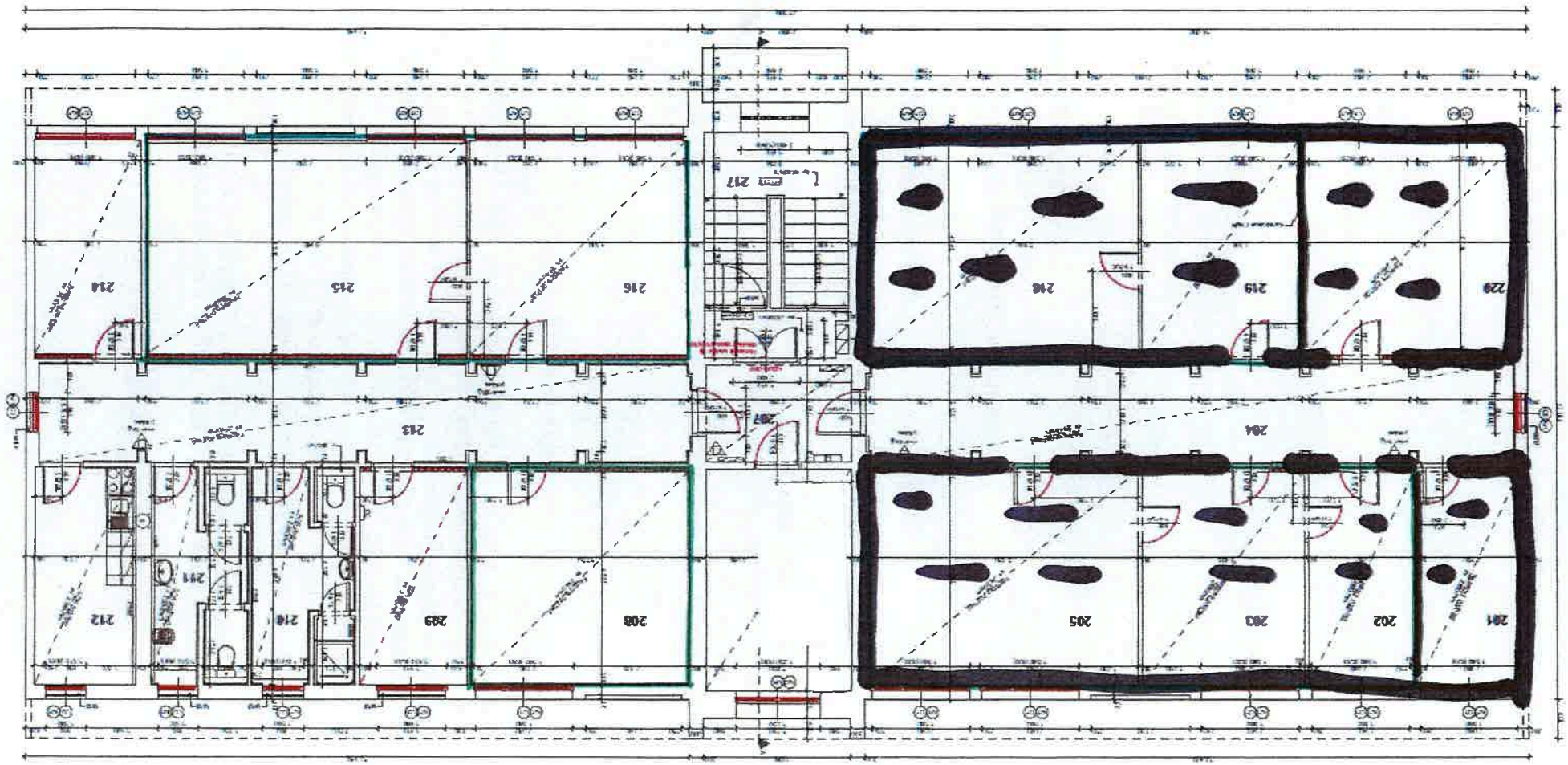
Podorys 2NP - nový stav, M 1:50
