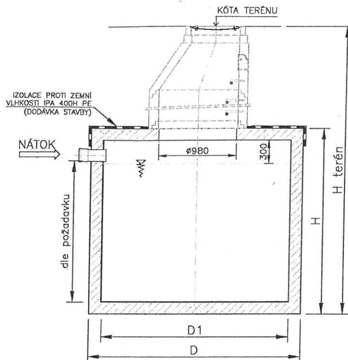
Obr. č. 5 - Rozměrové schéma typu PP nádrže válcové pro obetonování
