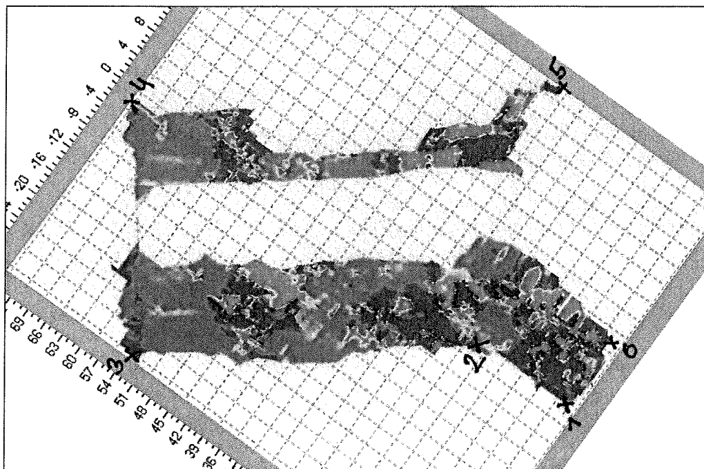
Obr.6 Výsledek měření pomocí magnetometrie s vyznačením rohových bodů budoucí haly
