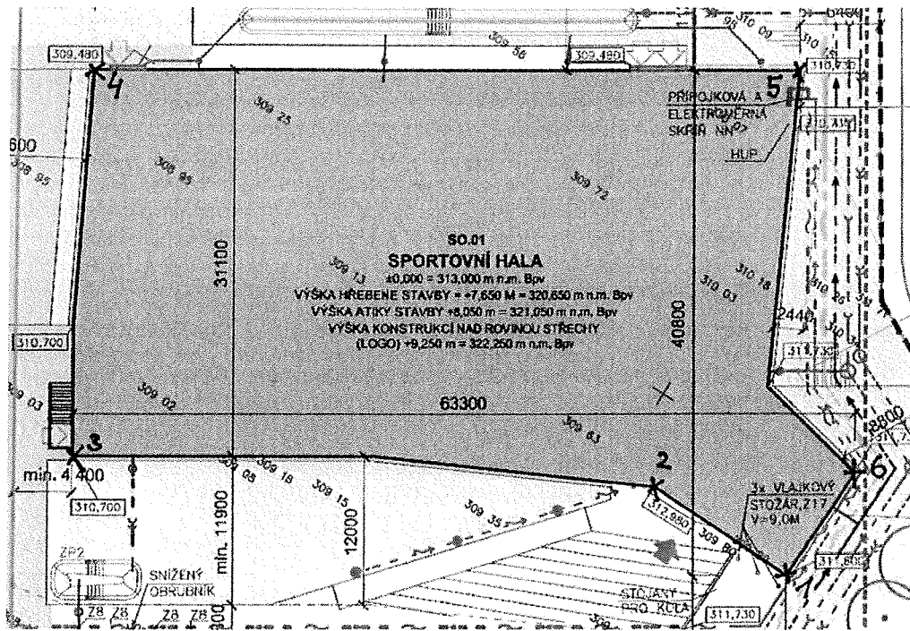
Obr.6 Půdorys haly s vyznačenými body, které byly využity při měření
