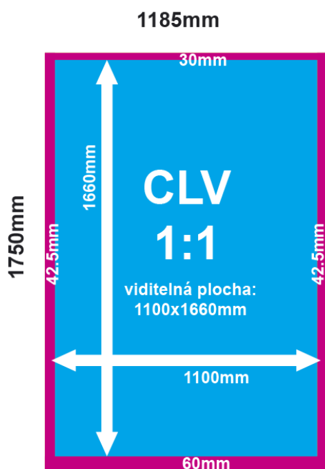
montáž 1:1
