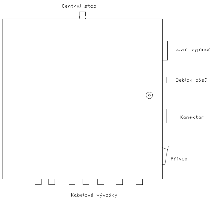
Obr. Rozvaděč – pohled
