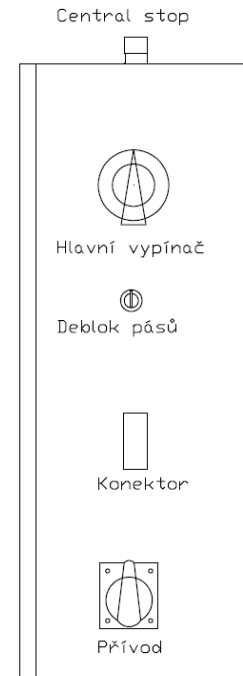
Obr. Ovládací prvky – rozvaděč
