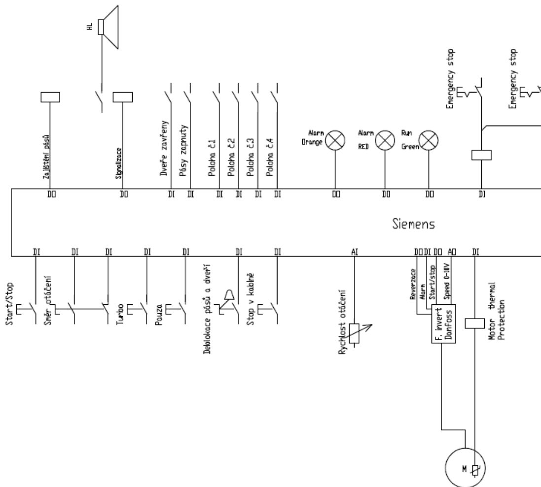
Obr. Schéma zapojení
