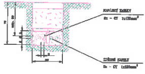
Vzorový řez trasou k napájecí NB 56C
