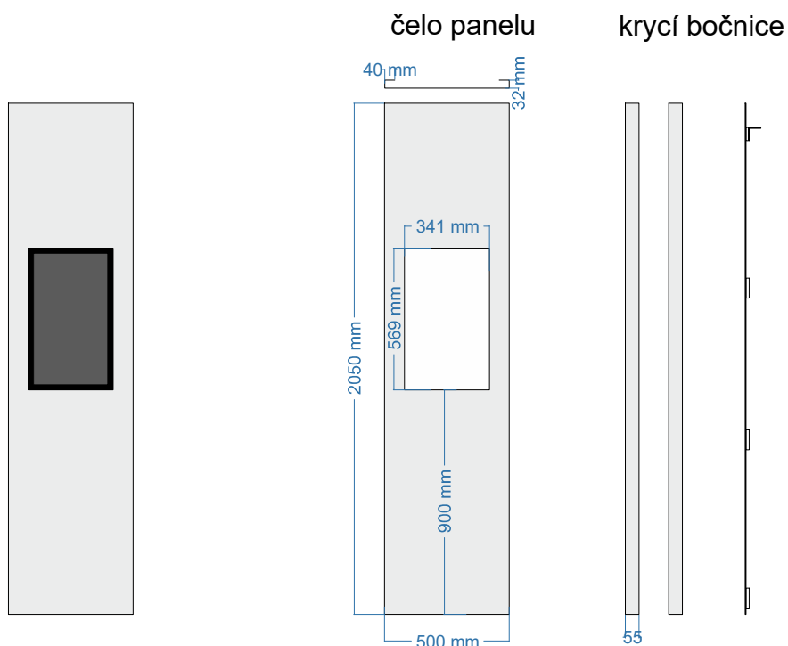
složený rám (kotvený rám, panel s nosnou mříží)
