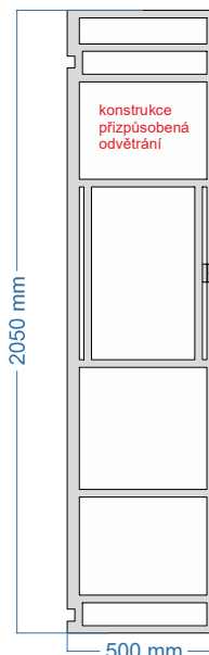
nosná mříž panelu
