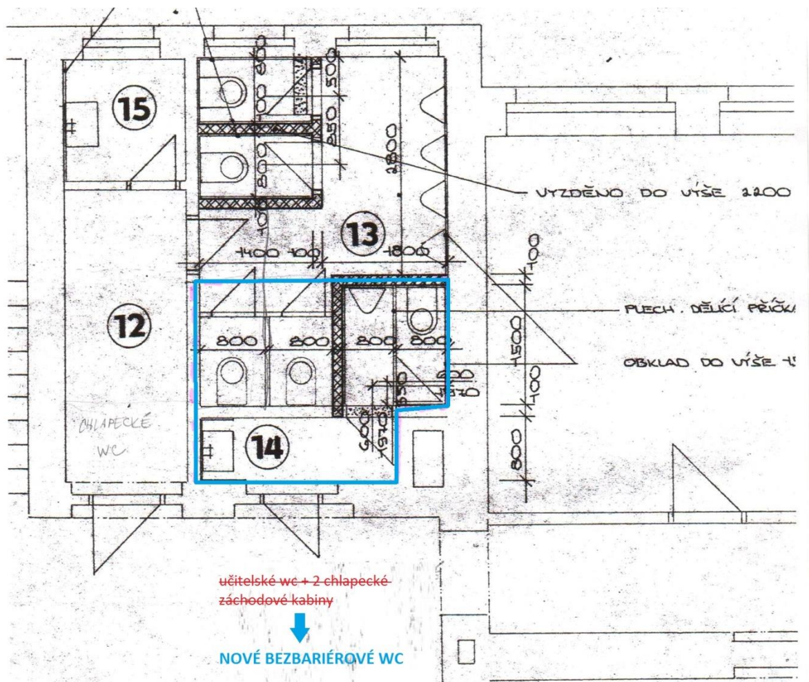
Schéma č. 2 – bezbariérové WC v 2.NP
