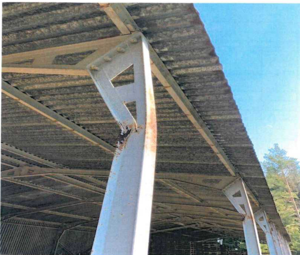
Fotografie č. 3: Detail narušeného nosníku.
