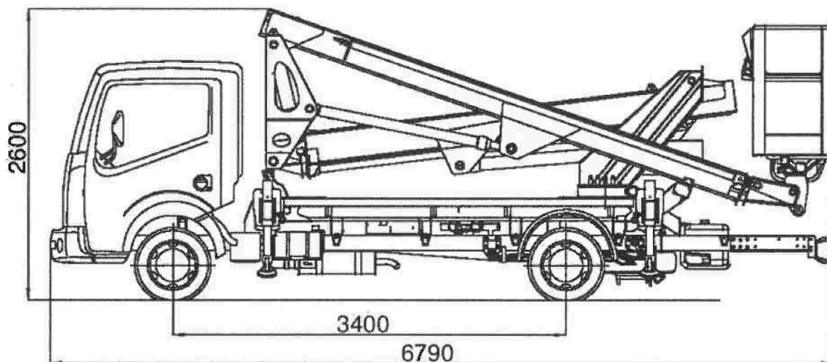
Obr. Rozměrový výkres plošiny na podvozku Nissan Cabstar
