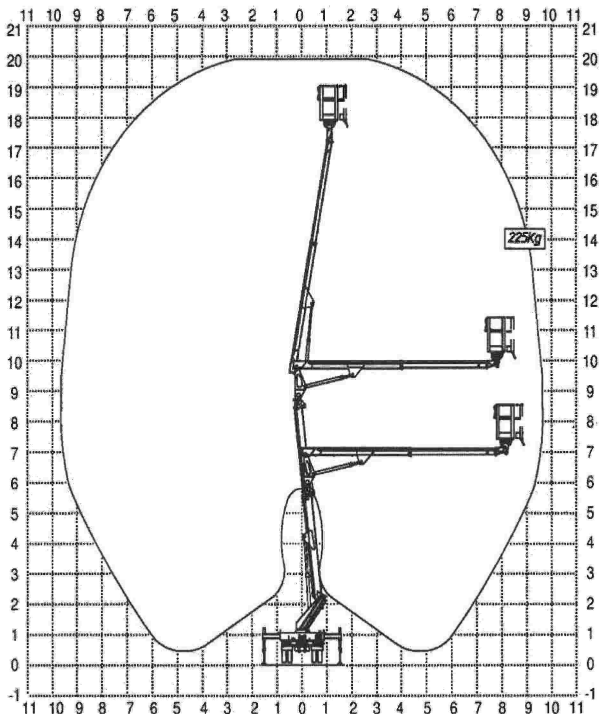
Obr. Pracovní diagram plošiny s podpěrami vysunutými do boku
