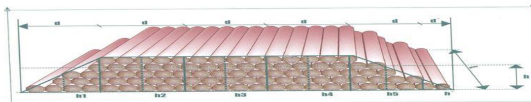
Obrázek č. 16: Princip měření dříví v hraních.
