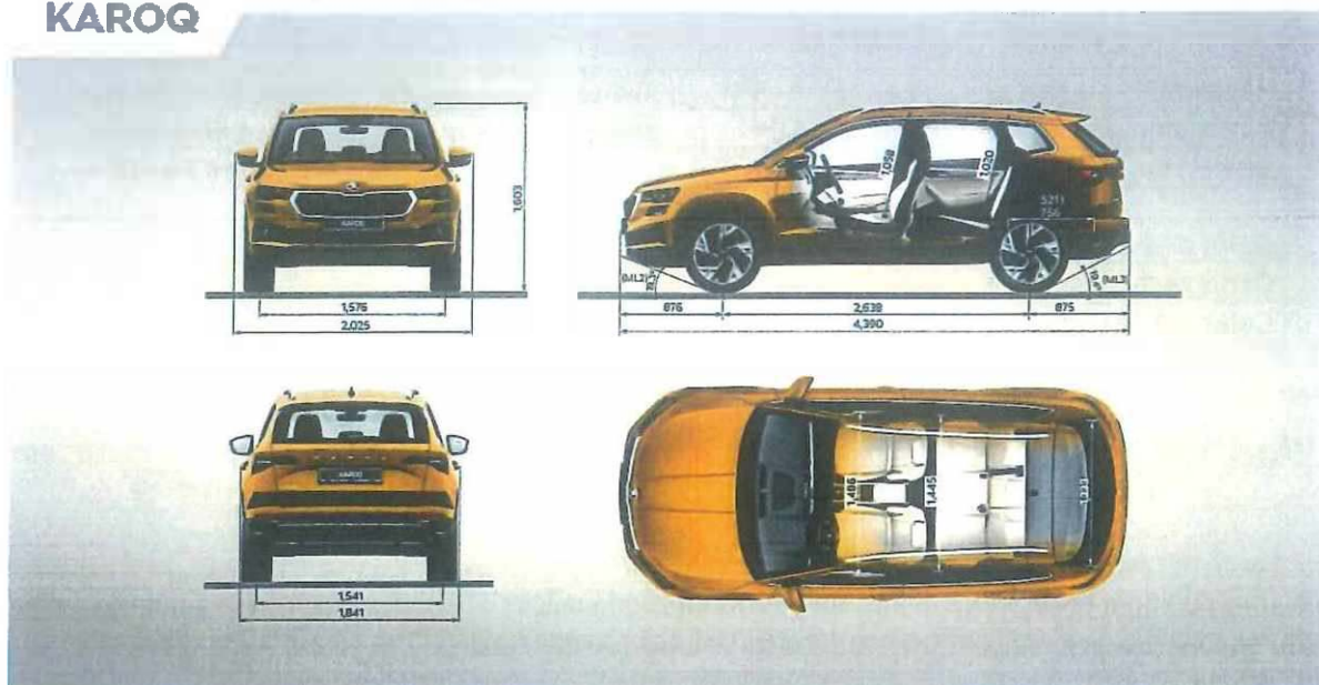
Rozměry nabízeného vozu
