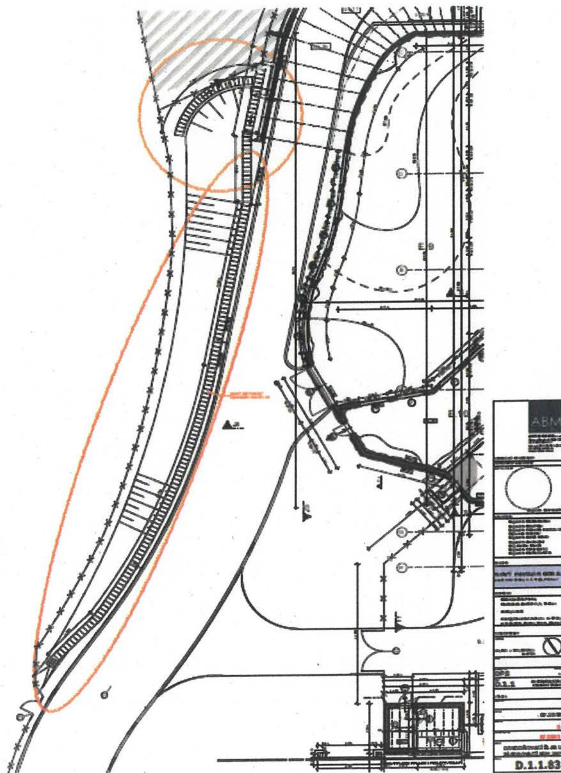
Příloha č. 1 - odvodňovací žlab u zásobovací komunikace 1.NP.
