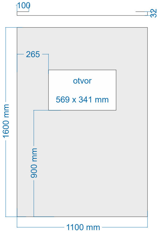
čelo panelu
