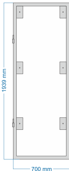
kotvený rám
