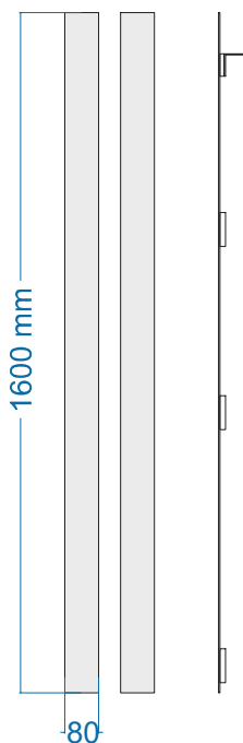
bočnice
