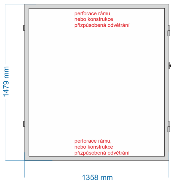
středový rám
