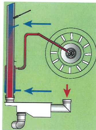
Multi Eco System: nástříkový systém výroby páry s tepelným výměníkem
