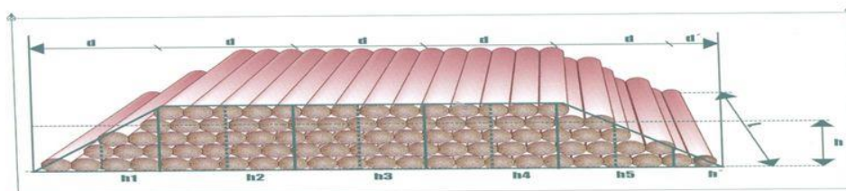
Obrázek č. 16: Princip měření dříví v hraních.
