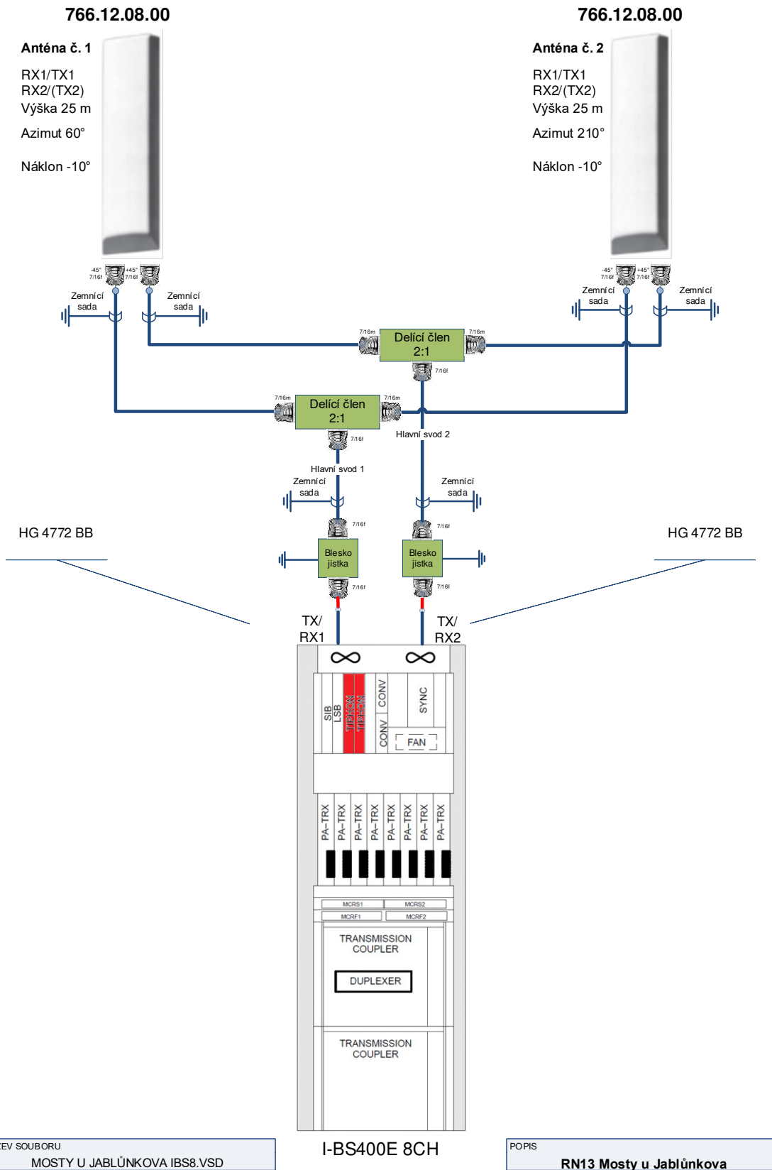
Obr. 6 Anténní systém PEGAS Mosty u Jablůnka
