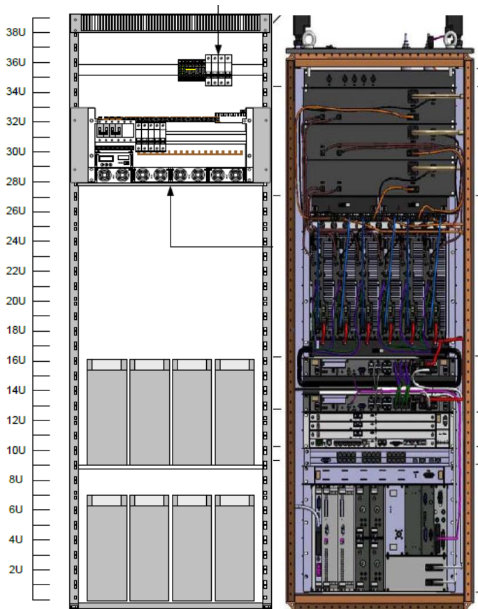
Obr. 3 sestava technologie
