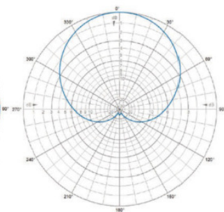
H-Plane | 425 MHz
