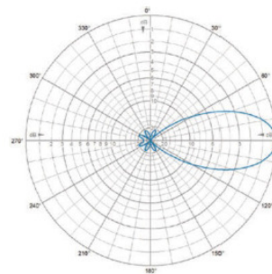
E-Plane | 425 MHz
