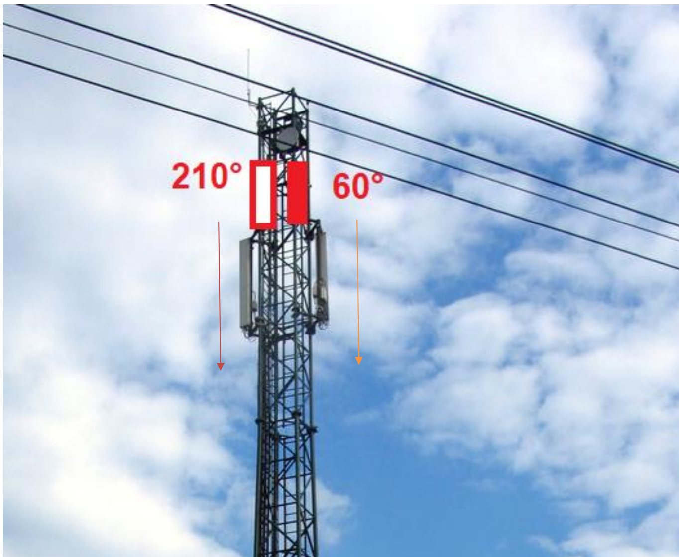
Obr. 5 Požadavek umístění antén na věži
