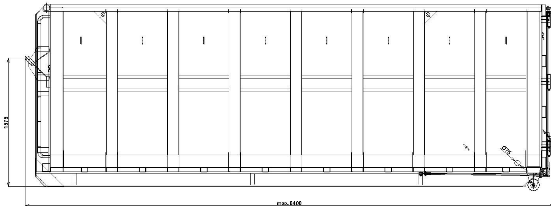
levá strana
