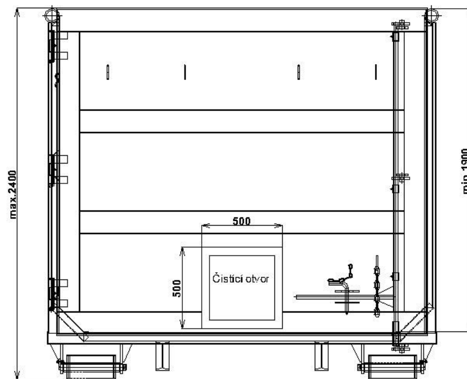
zadní pohled
