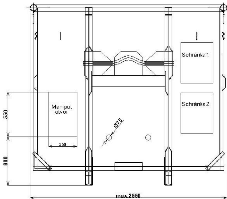
přední pohled
