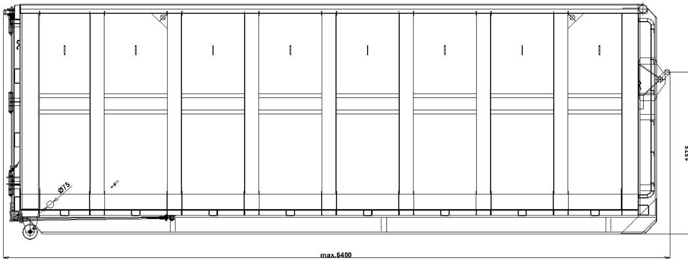
pravá strana
