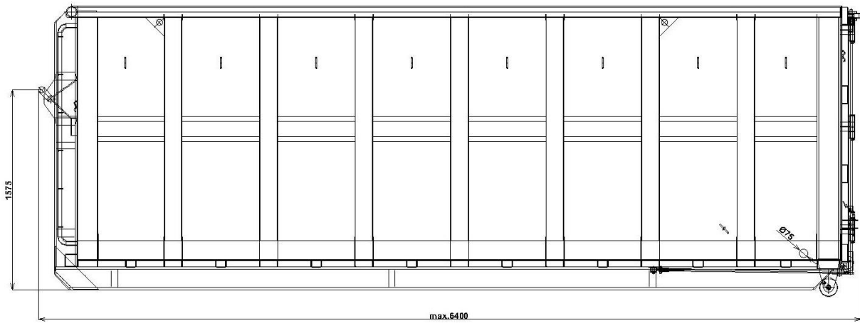
levá strana
