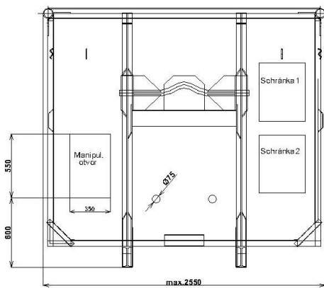
přední pohled
