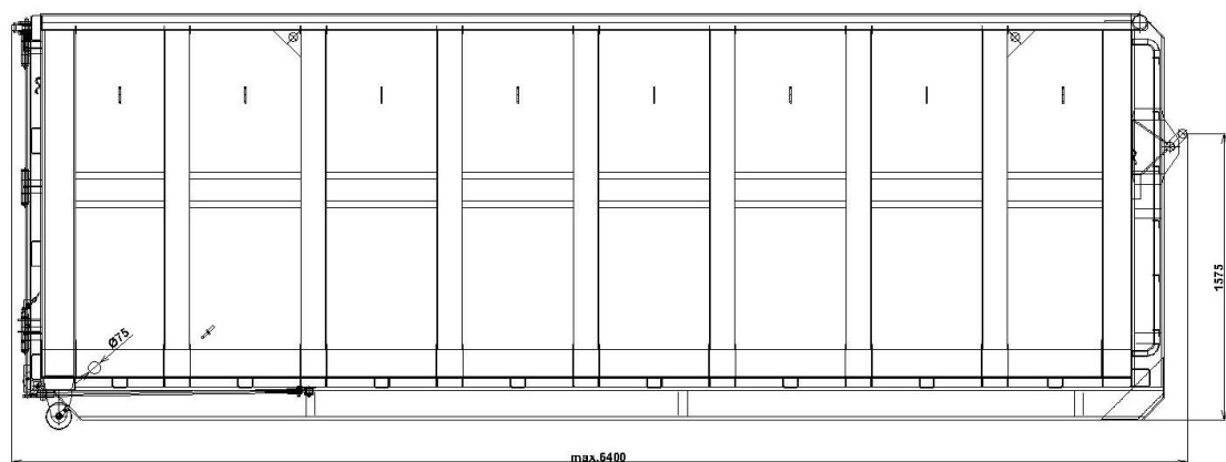
pravá strana
