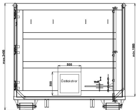
zadní pohled
