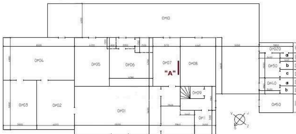
MNICHOVO HRADIŠTĚ - VÝPRAVNÍ BUDOVA - PŘÍZEMÍ KM 89,197 IC 5000002117
