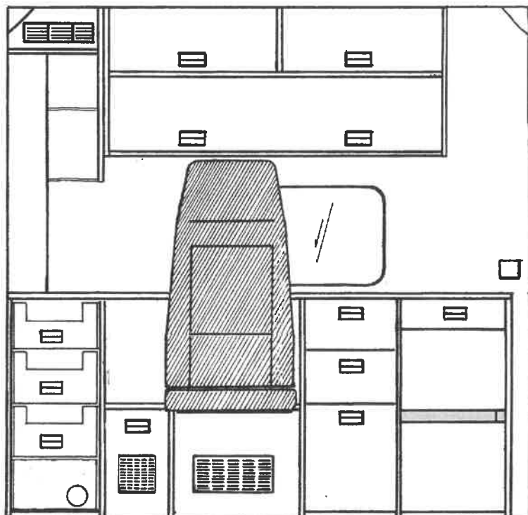
Schéma nábytkové zástavby vozidla - dělící přepážka:
