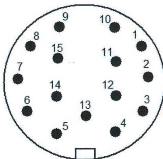
Obr.1-15 -pin zásuvka
