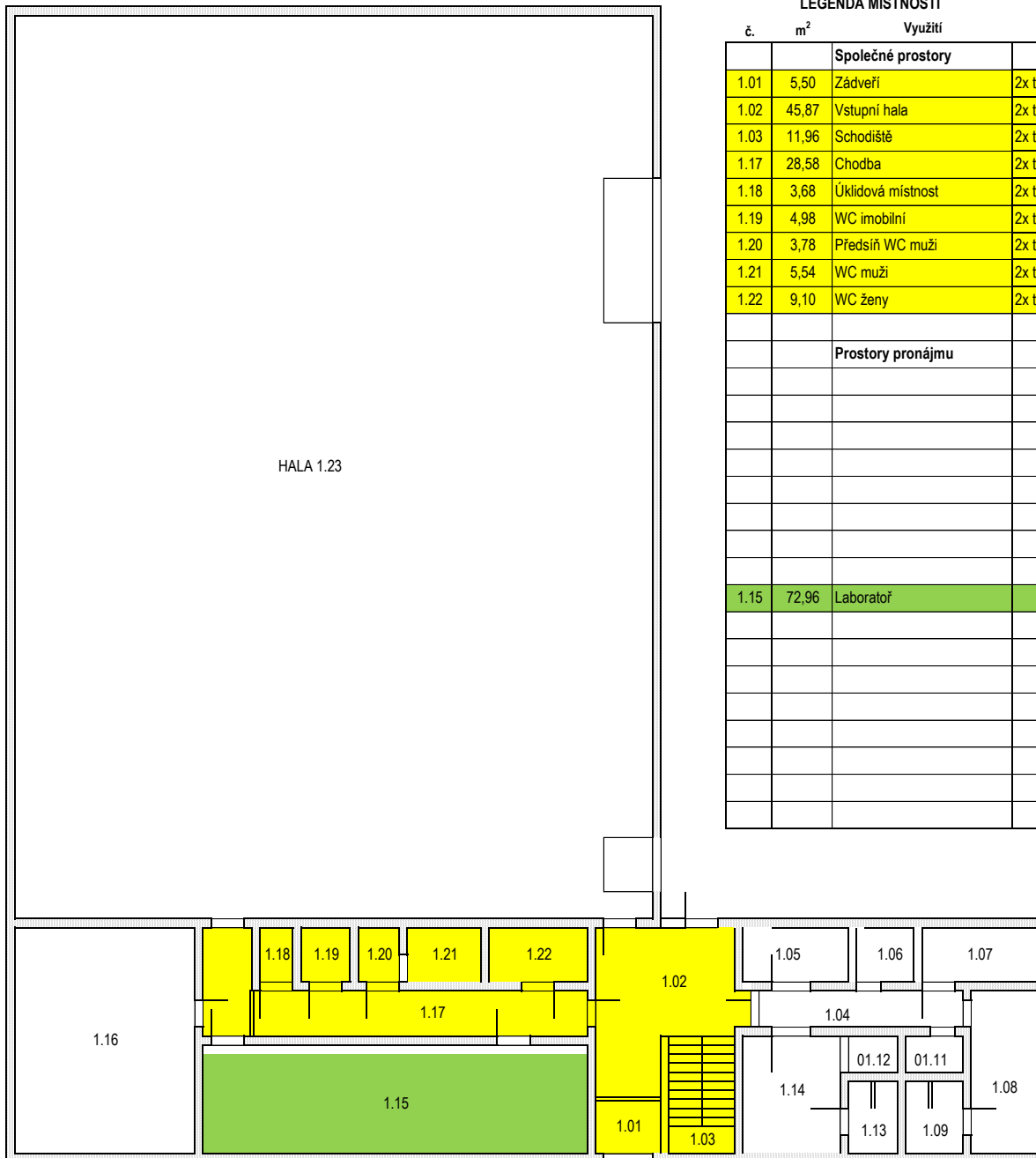
LEGENDA MÍSTNOSTÍ
