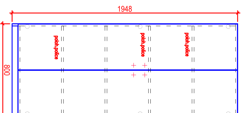
585 - skříň policová - 4 ks
