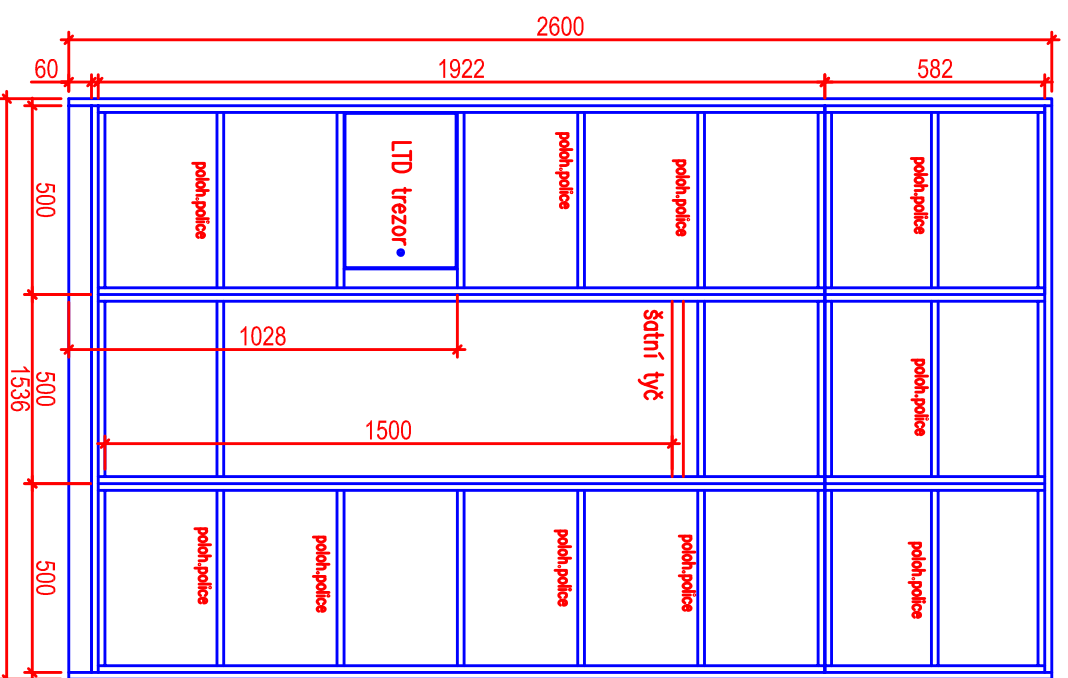
ŠS-PD - pohled bez dveří
