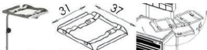
Nerez sklopný stolek - komplet rozměr stolku 49x35cm vpravo • sklopný stolek s prolisem 2 mm z nerez oceli AISI304; nosnost: 10 kg • u nízké verze vozíku nelze stolek kombinovat s jiným příslušenstvím na stejném boku vozíku
