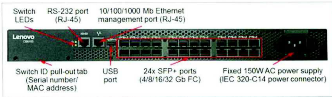
Obrázek 1 DB610S FC SAN Switch-Pohled na porty
